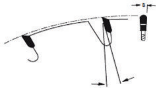
Zahnform = flach mit Fase (FF)
